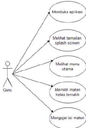
Gambar 2. Usecase Diagram Aplikasi Pembelajaran Berbasis Multimedia
