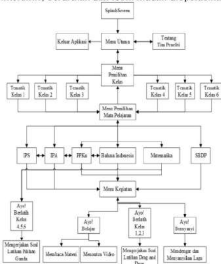
Gambar 14 Struktur Navigasi Aplikasi
